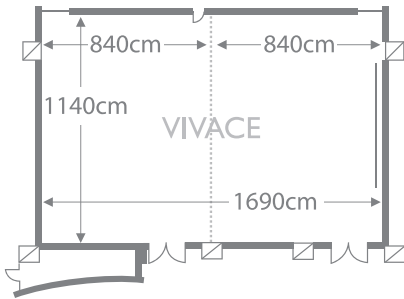
Height 400cm
