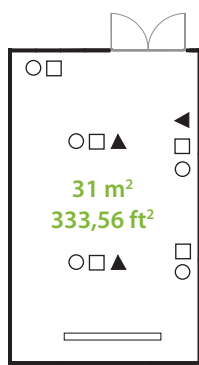
Orion
