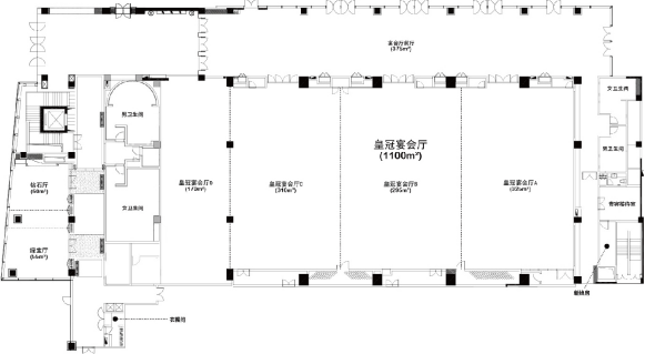
一层皇冠宴会厅平面图
